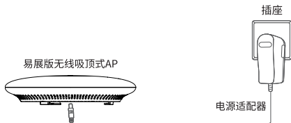
图2-2 DC供电示意图示
